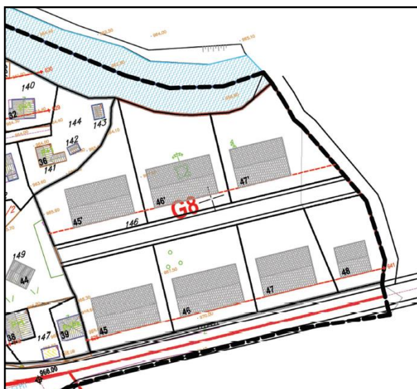
регулација и нивелација
